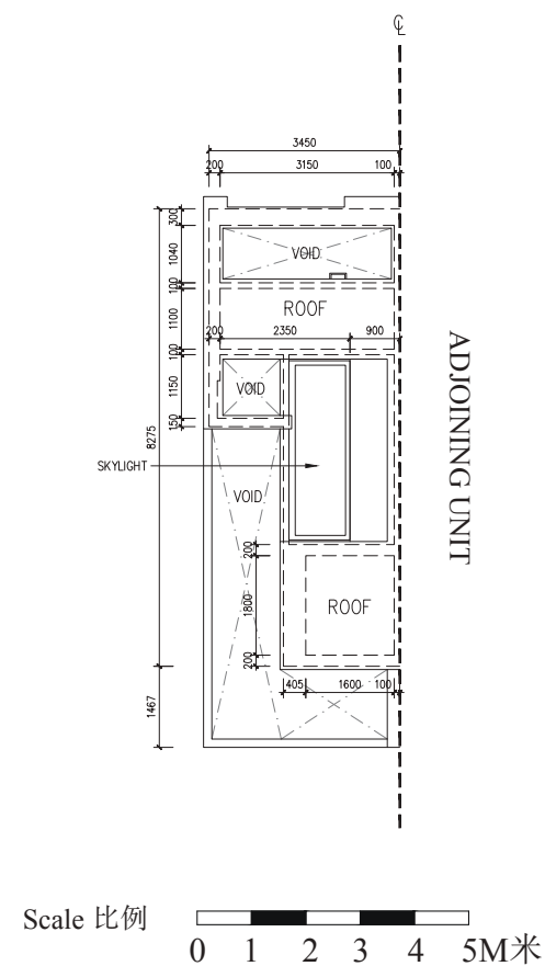
上層天台平面圖 Upper Roof Floor Plan
