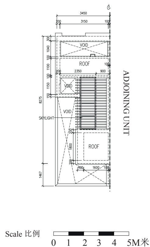
上層天台平面圖 Upper Roof Floor Plan
