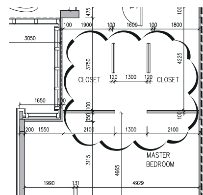
上層天台平面圖 Upper Roof Floor Plan
